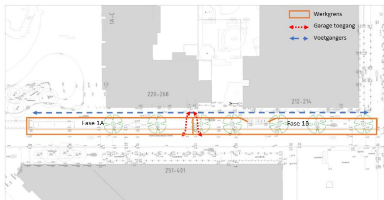
Afbeelding 1 fasering Gaasterlandstraat
